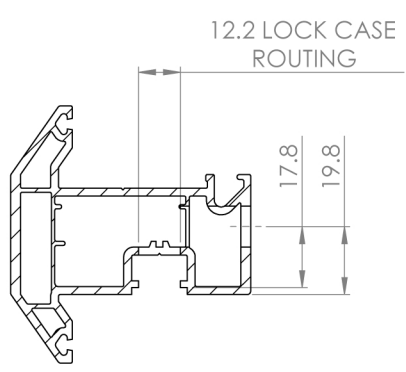
SECTION A-A SCALE 1 : 1.5
